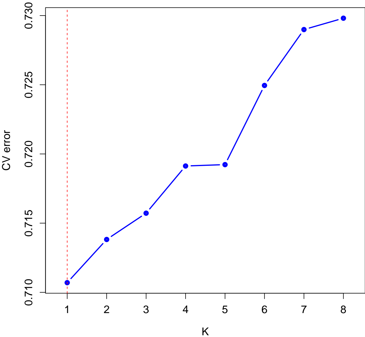
CV error
